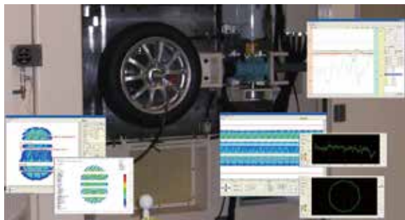
タイヤ試験機と解析ソフトウェア
